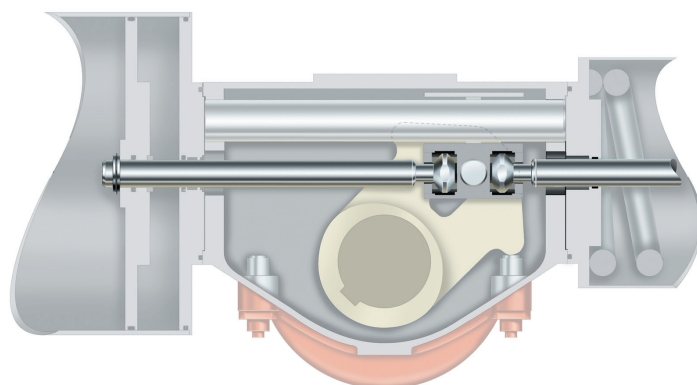
Powr-Swivl™
